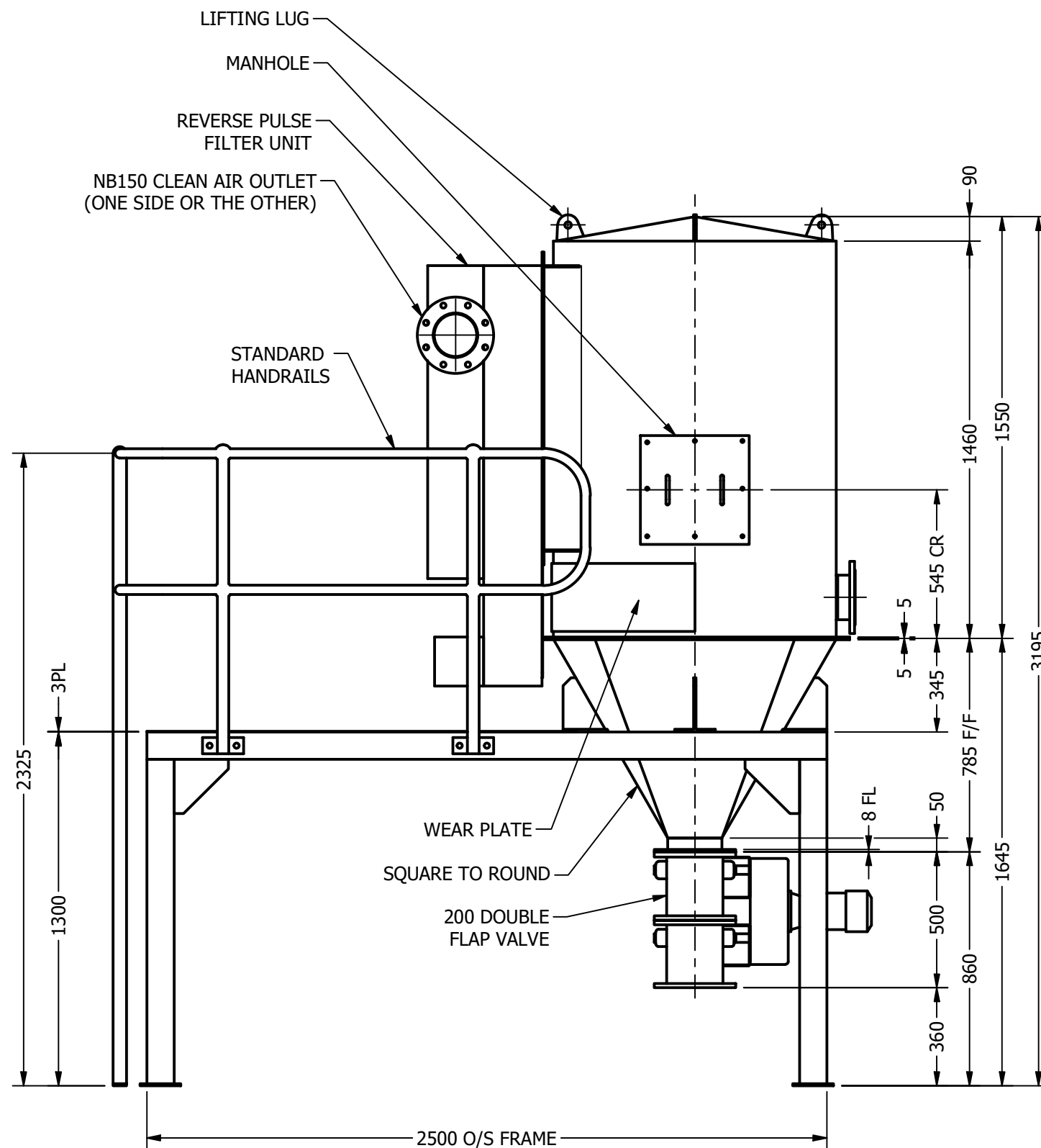
MANHOLE SIDE
